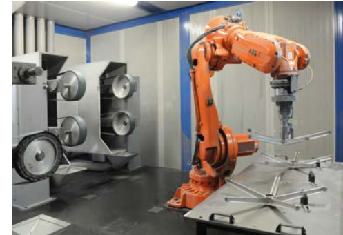
Τρόχιμα - Γυάλισμα με χρήση ρομπότ Sharpening - Polishing with the use of robotics
